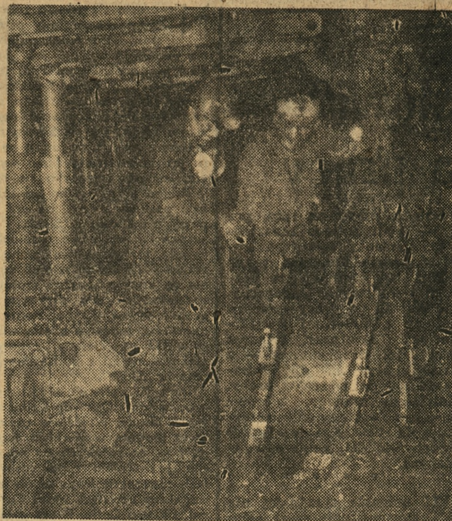
Ponad trzy czwarte węgla z przodków eksploatacyjnych wybiera się mechanicznie. W kopalniach pracuje 680 kombajnów, 41 strugów i 360 zespołów wręboladujących. Tadeusz Formela i Adam Zgolik z przodującego, VI oddziału kopalni „Knurow” przy kombajnie KB-125.
