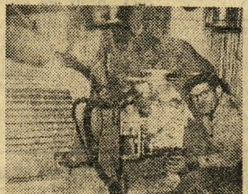
Na zdjęciu: brygada Wincentego Turka instaluje nową pompę zasilaającą w cukrowni szamotulskiej. Poniżej — Leon Kowal przy montażu nowej krajalnicy typu RK-13 w tej samej cukrowni.
