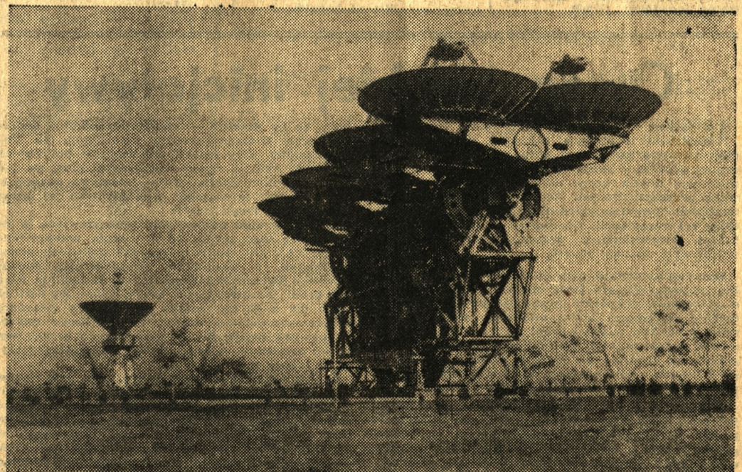
Olbrzymia antena znajdująca się w radzieckim ośrodku badań kosmicznych, która odbiera sygnały z Wenus IV, waży 1500 ton. Mimo swej wagi zespół może być nastawiany pod dowolnym kątem. Średnica jednego „talerza” wynosi 16 m.
