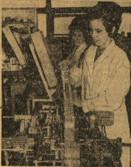
Agregat do obciążania baterii folią. Fot. — K. Przychodźki
