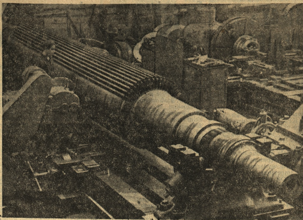
Na zdjęciu: rotor turbogeneratorsa o mocy 500.000 kW produkowany w leningradzkiej fabryce „Elektrosila”. CAF — Interpress
