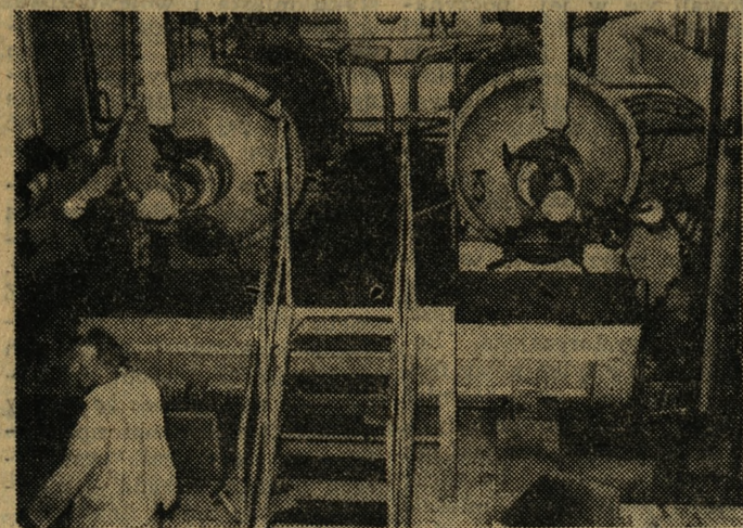
Oto część urządzeń aparatury Hartmanna, tak zwane destruktory, w których pod wysokim ciśnieniem gotuje się surowiec mięsny na mączkę.
