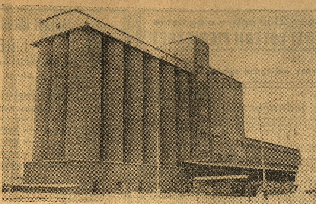
Tak wygląda z zewnątrz Wytwórnia Pasz w Kaliszu...
