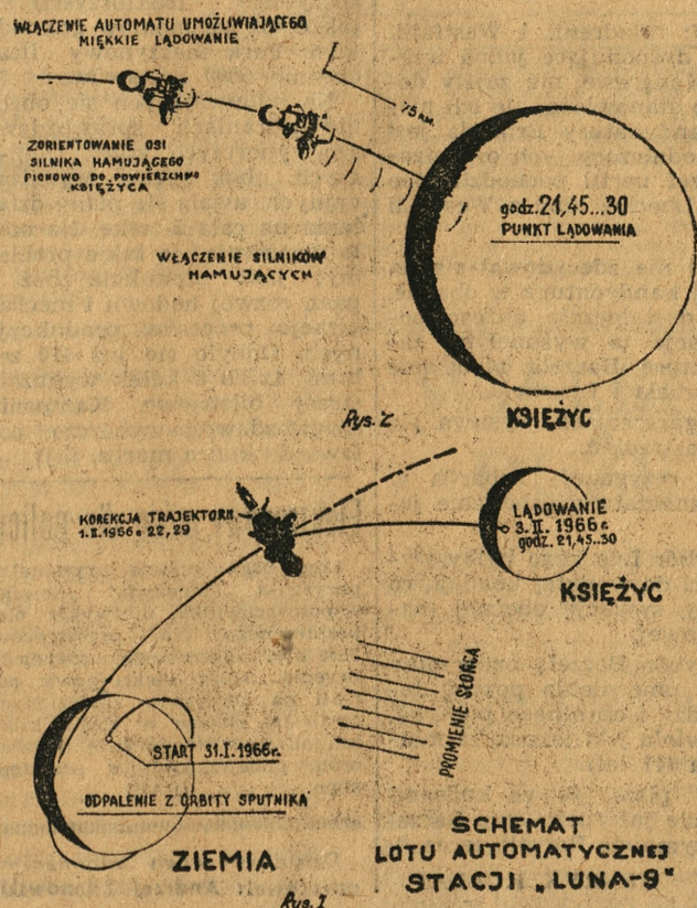
SCHEMAT LOTU AUTOMATYCZNEJ STACJI „LUNA-9” NA ODCINKU HAMOWANIA 3.1966.
