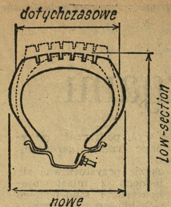
Tak mniej więcej wygląda różnica między dotychczasowym kształtem opon (zaznaczone linią przerywaną) a nowym typem Law Section, produkowanych przez firmę Pneumant.
