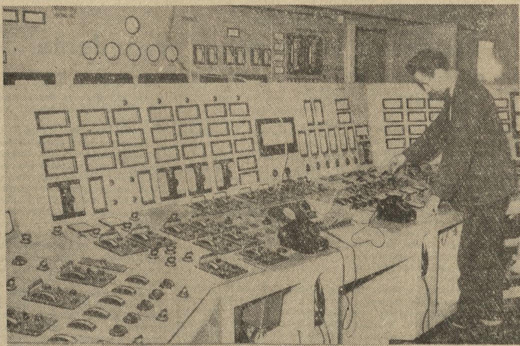
Na zdjęciu — pulpit automatycznego sterowania turbozespołem 125 MW. Stąd za pociśnięciem guzików i dźwigni reguluje się pracę kotłów parowych, podajników węglowych, turbiny. Fot. — K. Przychodzki
