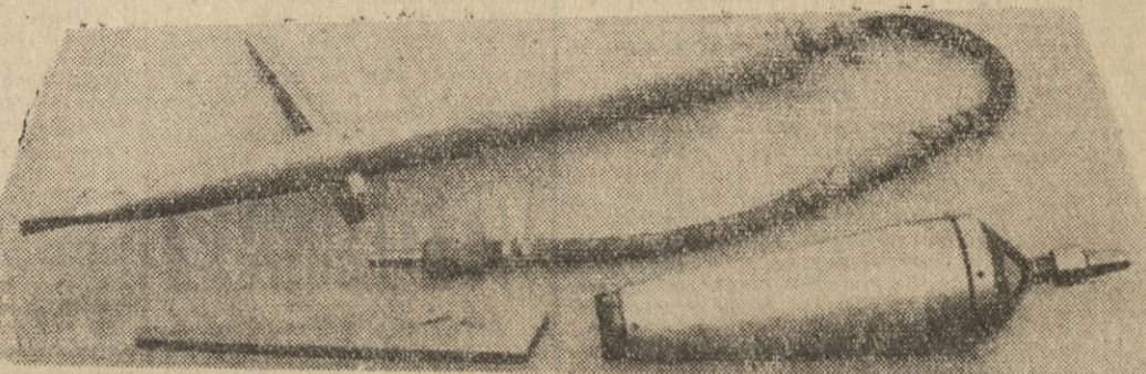
Przyrząd do przebijania gruntu KRET typ 88ZD z wyposażeniem
