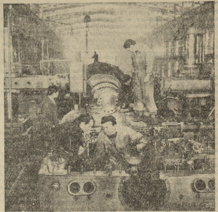
Komisja techniczna rozpoczęła w zakładach im. Gen. Świerczewskiego w Elblągu odbiór największej z budowanych dotychczas w Polsce turbiny elektrycznej o mocy 120 megawatów. Turbina ta przeznaczona jest dla elektrowni w Koninie. Na zdjęciu: fragment ostatnich prac montażowych przy turbinie o mocy 120 MW.
