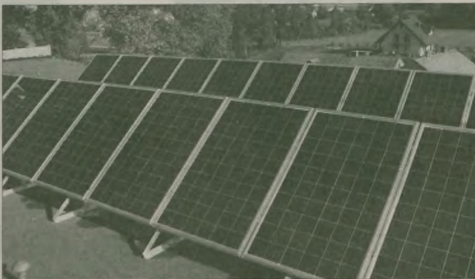
Panele fotowoltaiczne na dachu budynku Urzędu Gminy w Przykonie.
