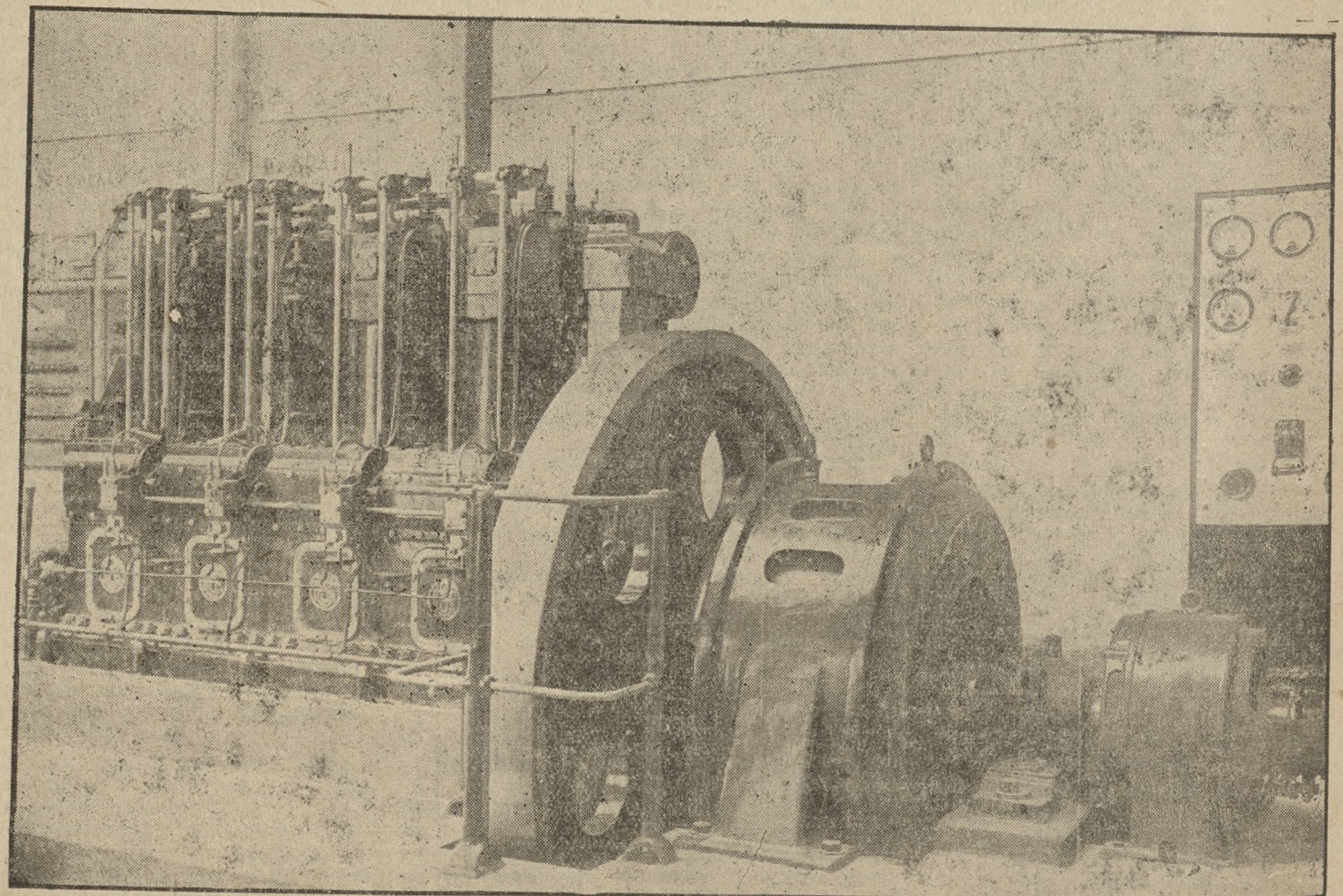
Duży silnik Diesla bezsprężarkowy, wykonany przez fabrykę „Ursus”. Typ ten nadaje się specjalnie dla browarów, gorzeln i małych elektrowni.
