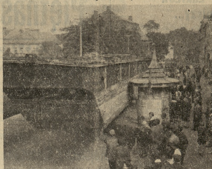
Krakowska ekspozycja Państwowej Komunikacji Samochodowej podjęła się trudnego zadania — przewiezienia poglobiarki rzecznej z Krakowa do Starego Sącza na Dunajec. Poglobiarka waży 60 ton, ma długości 27 m i szerokości 7 m. Na specjalnych przyczepach, które ciągnęły dwie ciężarówki „Tatra”, poglobiarka została przetransportowana drogą lądową. Najcięższe były przejazdy przez miasta zwłaszcza na wąskich ciasnych uliczkach.
