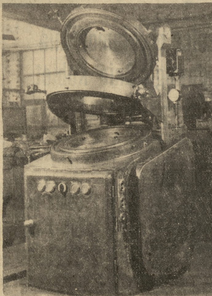
Prasa piętrowa do wulkanizacji opon rowerowych (otwarta). Fot. — A. Zwierski
