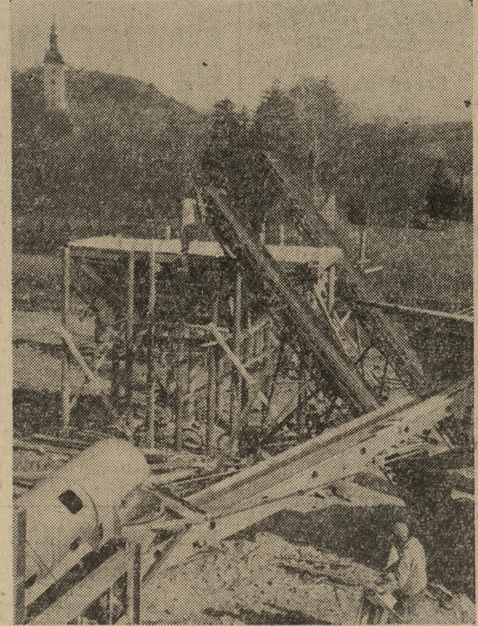
W celu zapewnienia dostatecznej ilości wody dla budującej się elektrowni w Turowie budujemy zapórę wodną na rzece Wilce k/Radomierzyc (pow. Zgorzelec).
