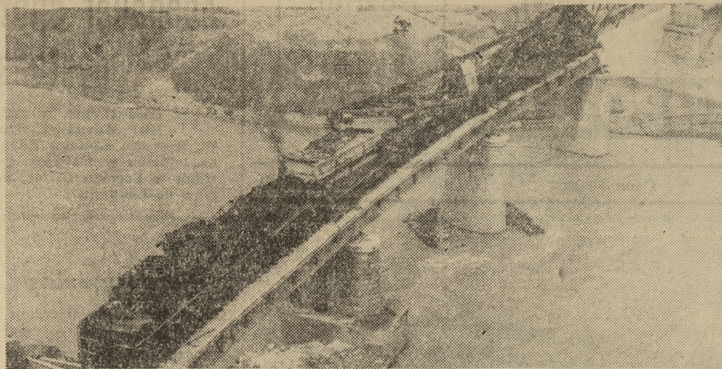
Na trasie Lanczhou-Chinghai (Wyżyna Tybetańska) buduje się most na rzece Huangshui. Na zdjęciu: Montaż przęsła mostu. Fot. — CAF
