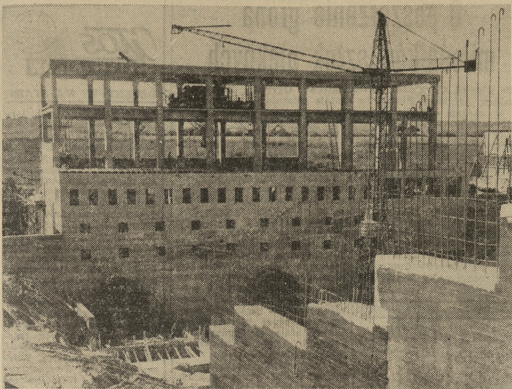
Fragment budowy siłowni w Koronowie.
