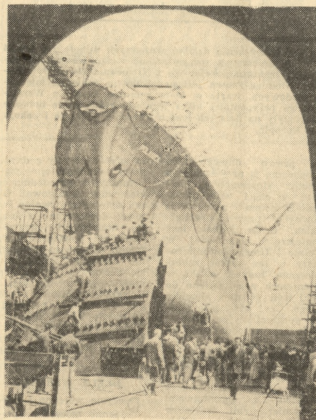
„Polanica” z nowej serii 6-tysięczników przed wodocieżnią. Fot. (2) „Głos”
