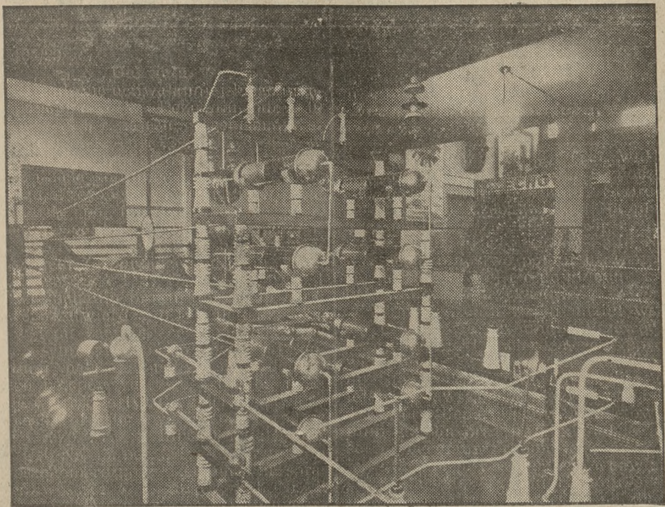
Laboratorium do badania wytrzymałości izolatorów; napięcie do 500 000 wolt. Ekspozat elektrowni Gródek.
