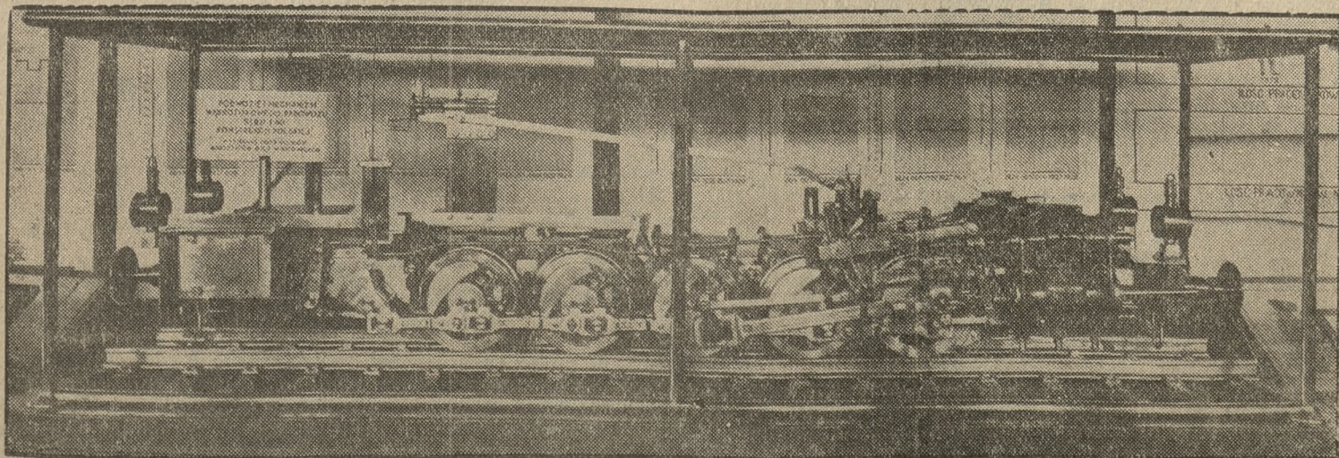
Podwozie i mechanizm wąskotorowego parowozu, konstrukcji polskiej; model wyk. uczn. warszt. D. K. P. Katowice
