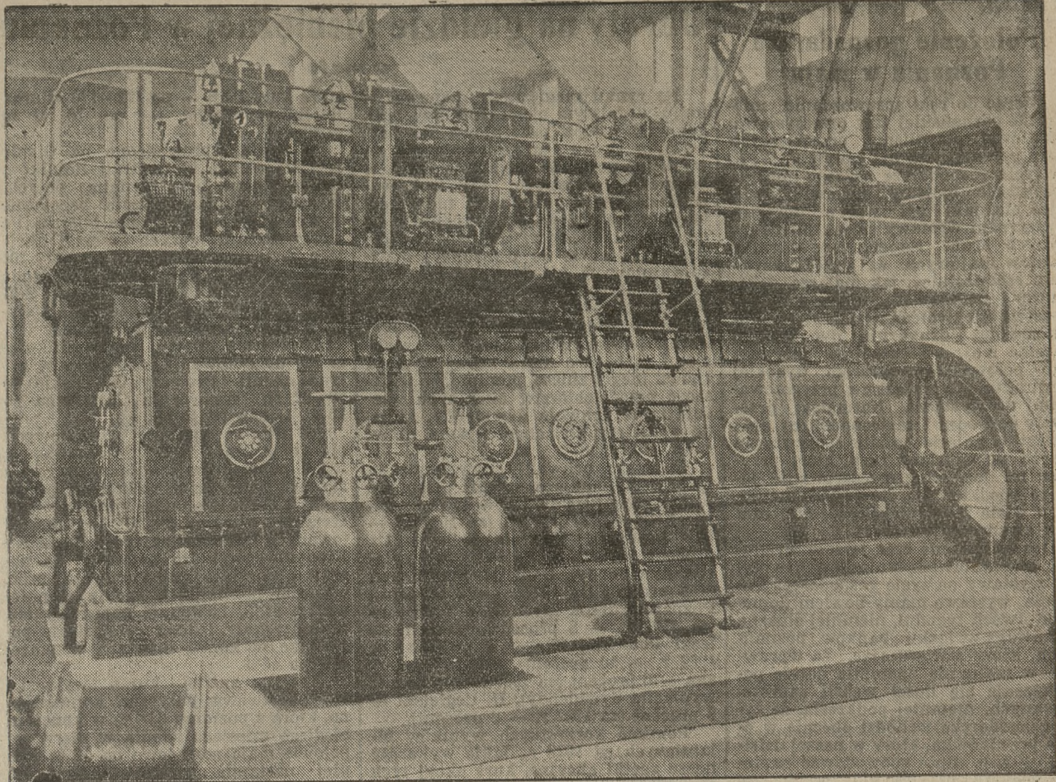
800-konny motor dieslowski w hali ciężkiego przemysłu.
