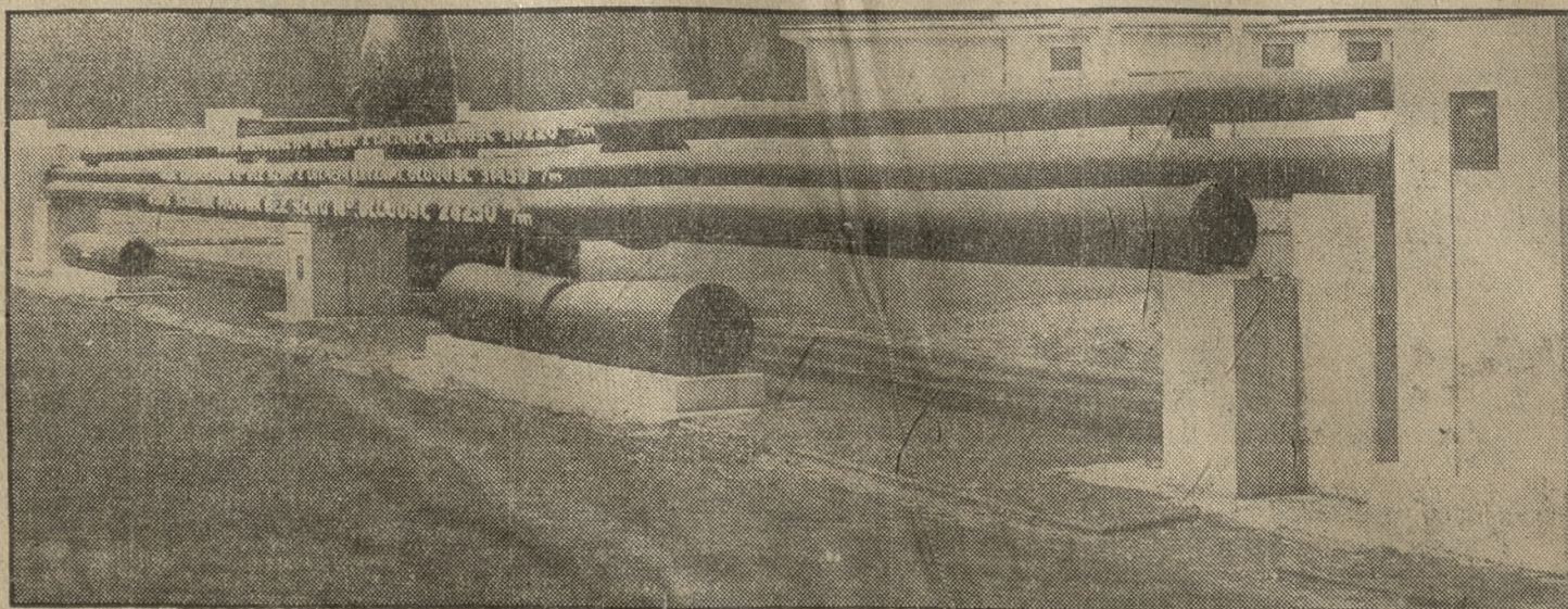
Stalowe rury bez szwu, długie na 28,50 i 31 metrów. Ekspozyty Huty Bismarcka.
