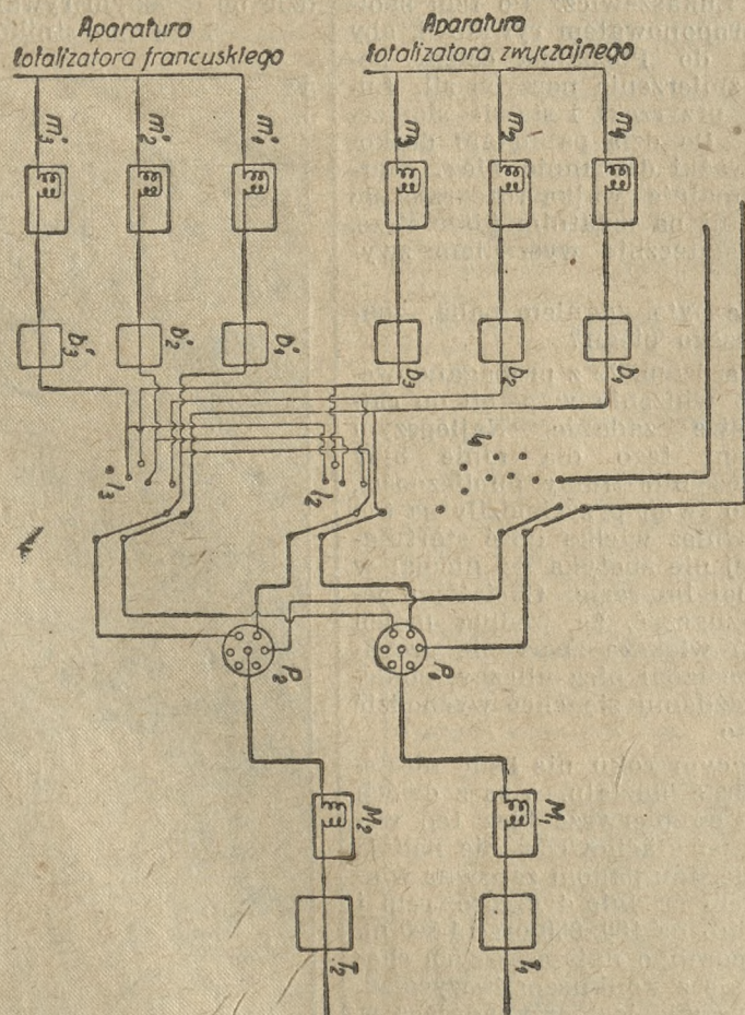
Schemat całej instalacji.
