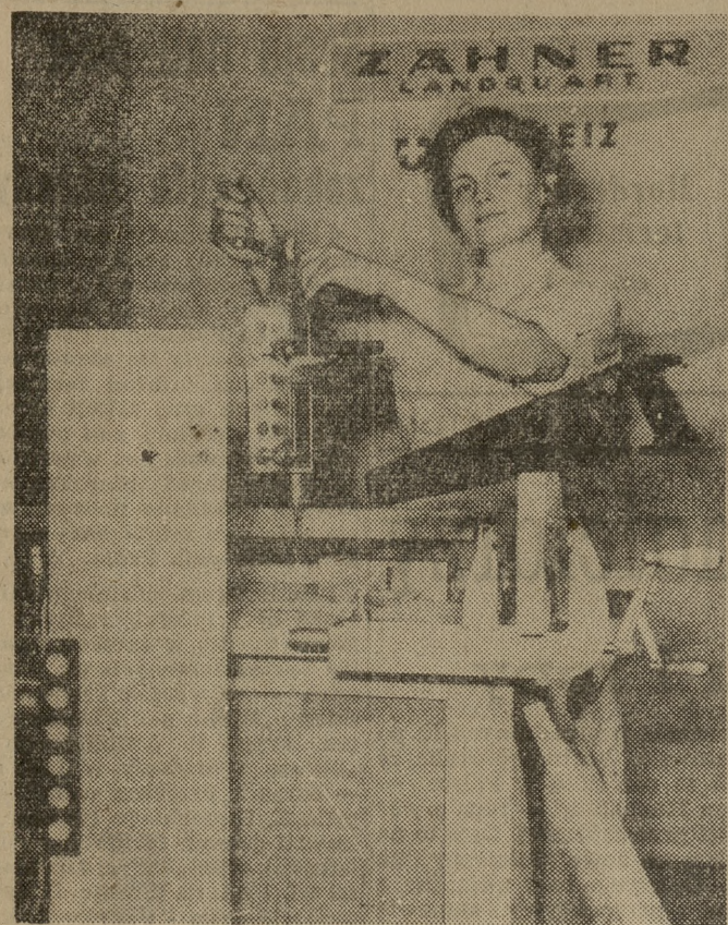
Warsztat stolarski, ważący tylko 3,5 kg, wyprodukowano w NRF. Na warsztacie tym można wykonywać wszystkie podstawowe prace stolarskie.
