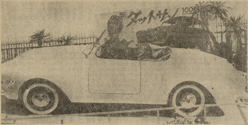
Zakłady Niosan wyprodukowały po raz pierwszy prototyp 4-osobowego samochodu sportowego o karoserii z plastiku. „Datsun 1000” posiada silnik 4-cylindrowy (988 ccm) o mocy 34 HP. Szybkość maksymalna 95 km/godz. Podwozie waży 510 kg, cały samochód — 1145 kg. Zużycie paliwa — 1 litr na 18 km. Nowy typ samochodu, zaprezentowany niedawno na wystawie tokijskiej, będzie produkowany masowo w przyszłym roku.
