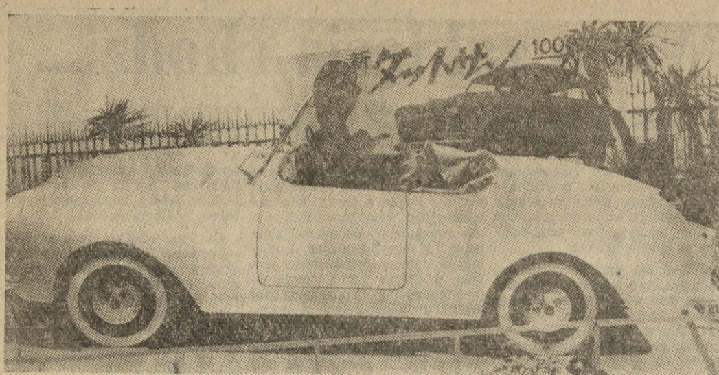
Zakłady Nisan wyprodukowały po raz pierwszy prototyp 4-osobowego samochodu sportowego o karoserii z plastiku. „Datsun 1000” posiada silnik 4-cylindrowy (988 cm) o mocy 34 HP. Szybkość maksymalna 95 km/godz. Podwozie waży 510 kg, cały samochód — 1145 kg. Zużycie paliwa — 1 litr na 18 km. Nowy typ samochodu, zaprezentowany niedawno na wystawie tokijskiej, będzie produkowany masowo w przyszłym roku.
