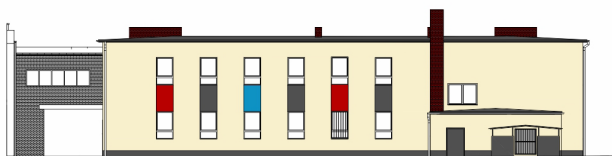
ELEWACJA PÓŁNOCNO-ZACHODNIA
