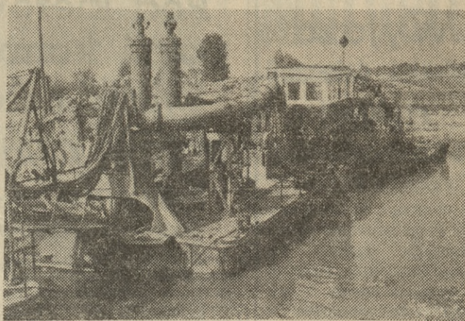
Pogłębiarka Smok III pracuje przy budowie kanału na odcinku Żerań—Zegrze. CAF — Fot. Mottl
