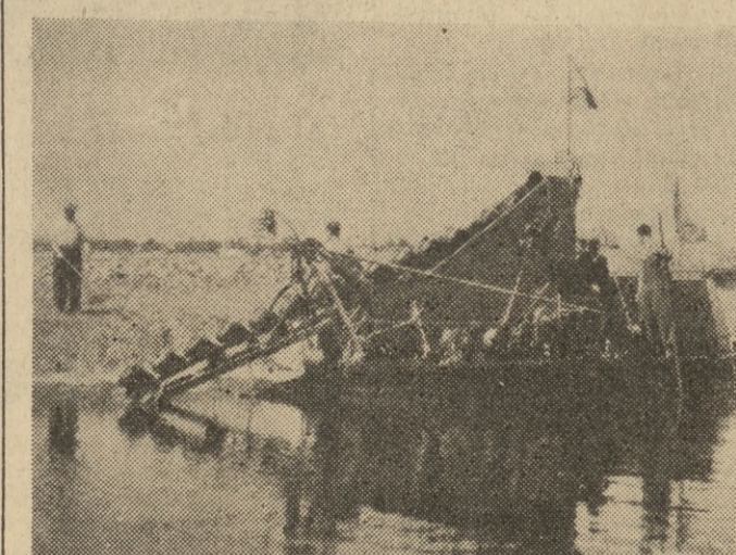
Na terenie powiatu Elbląg zakończono próby prototypu pogłębiarki kanałów i rzek, prowadzone przez Zarząd Wodno-Melioracyjny w Gdańsku. Nowy typ pogłębiarki, która zastępuje pracę ręczną 15 ludzi, zdał całkowicie egzamin.
