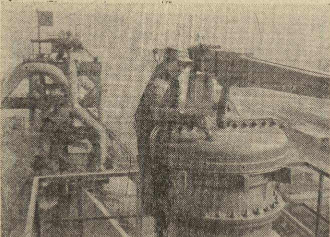
Niedługo już ruszy także wielki piec nr II w Hucie im. Lenina. Obecnie trwają intensywne prace nad wykańczaniem poszczególnych obiektów tego pieca ważącego „tylko” 55 ton.
