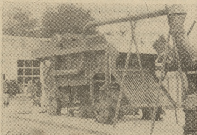
Dołą pomocą dla wsi są nowoczesne wydajne w pracy maszyny rolnicze. Te potężne młocarnie szerokomłotną, czyszczącą — MSC-15, wykonała Huta Stalowa Wola. Maszyna młoci i czyści 2 tony ziarna na godzinę.
