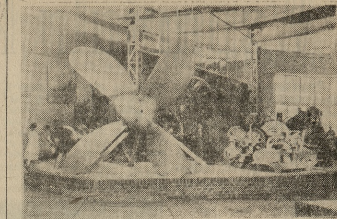
Porównajcie wielkość człowieka z tym eksponatem naszego przemysłu okrętowego. Jest to śruba napędowa statku o ciężarze 4700 kg dla rudowęglowca 5000 TDW.
