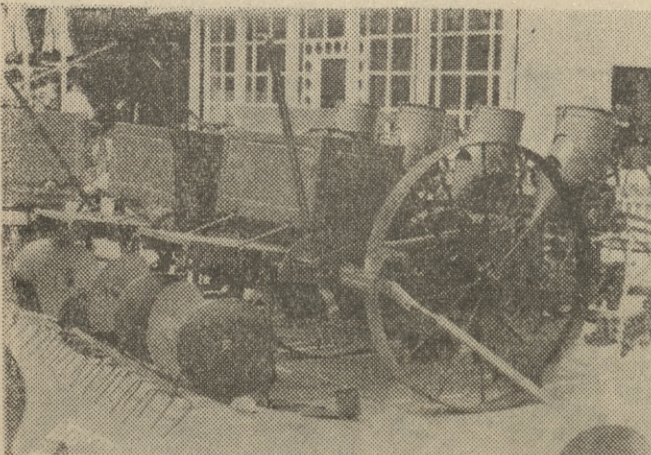
Wśród prototypów maszyn rolniczych znajdujemy na Targach sadzarkę krzyżowo-gniazdzową SKG-4. Sadzarka o wydajności 6 hektarów dziennie, zaoszczędza 5 dniówek na 1 hektar w stosunku do pracy ręcznej.
