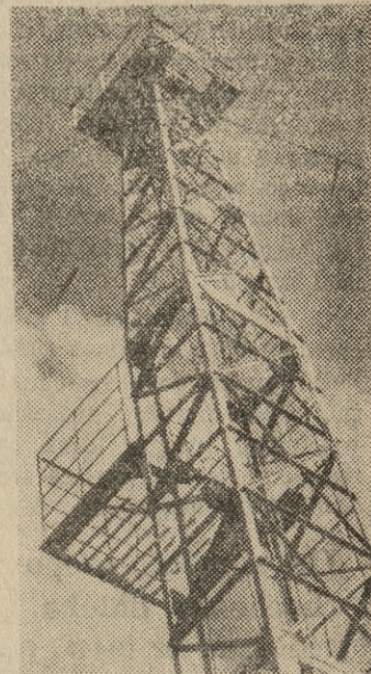
Wieża zespołu wiertniczego „JL-35“, przeznaczona do wiercenia metodą obrotową do głębokości 1500 m. Ciężar zespołu 75 000 kg.
