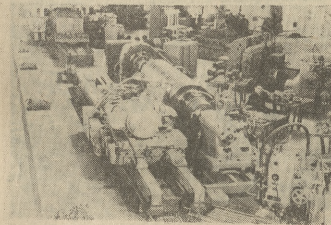
Z dumą możemy stwierdzić, że wiele naszych maszyn nie ustępuje zagranicznym. Oto jedna z tego rodzaju maszyn — szlifarka do wałów hutniczych SHA-90. Służy ona do walcowego wkleśnięcia i wypukłego szlifowania i polerowania wałców hutniczych.
