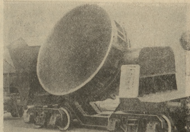
Polskie fabryki wystawiły na Targach doskonale skonstruowane i wykonane lokomotywy i wagony. Oto jeden z nich — kadź żużlowa wykonana przez Hutę im. Nowotki w Ostrowcu Kiel. Pojemność kadzi — 10,9 m 3 , ciężar wagonu 50,2 tony.
