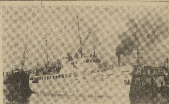
W stoczni im. Gheorghiu-Dej w Budapeszcie został spuszczonej na wodę nowoczesny statek „Mazowsze“ przeznaczony dla Polski. Długość jego wynosi 65 m a szerokość 9 m. Statek może zabrać 600 pasażerów. Na zdjęciu: statek „Mazowsze“ w stoczni budapeszteńskiej.
