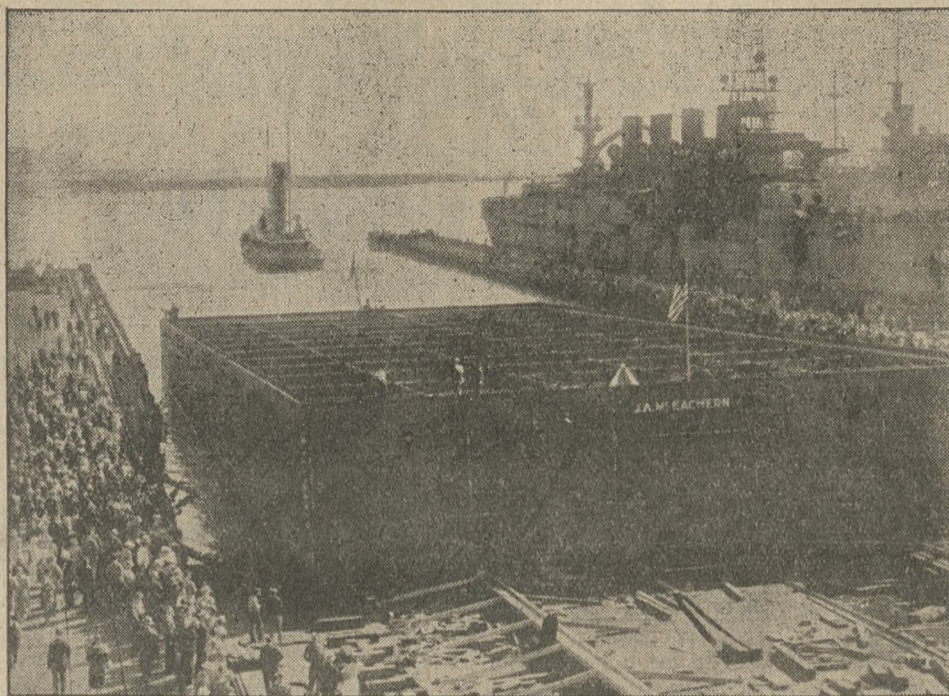
Uwidoczniony na powyższej fotografii największy keson na świecie użyty został do budowy olbrzymiego mostu pomiędzy San Francisco i Oakland w Kalifornii. Keson ten ma 66 mtr. długości i 32 mtr. szerokości.
