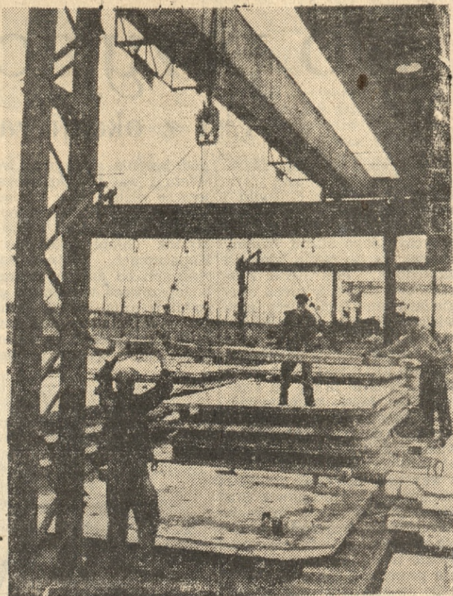
CAF — fot. Dąbrowiecki Fragment Bazy Zaopatrzeniowej Palacu Kultury i Nauki na Jelonkach — płyty stropowe przygotowane do transportu na budowę. Płyty tego rodzaju coraz częściej stosuje się na polskich budowach.
