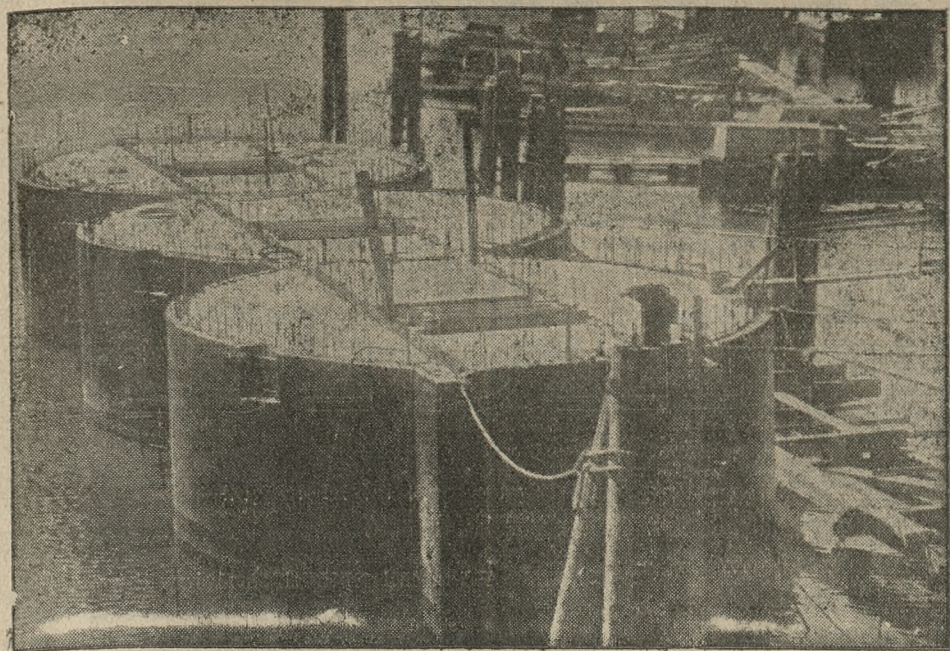
piwające fundamenty betonowe. Oto trzy z liczby 20 kesonów ze stali i betonu, które przetransportowano morzem na przestrzeni 65 km. do Santa Monica (Kalifornia). Kesonu te użyte będą jako łamacze fal w nowym porcie jachtowym.
