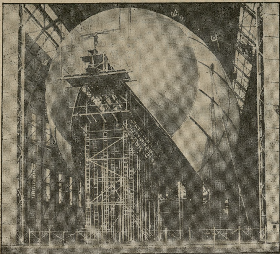
Budowa nowego niemieckiego statku nap. wietrznego L Z 129 zbliża się ku końcowi. Zdjęcie nasze przedstawia właśnie chwilę pokrywania oponą olbrzymiego kadłuba. Nowy ten „Zeppelin” przeznaczony jest tymczasowo na służbę transatlantycką pomiędzy Niemcami a Stanami Zjednoczonymi A. P.
