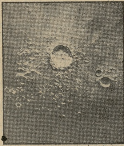
Pierścień Kopernika na Księżycu.
