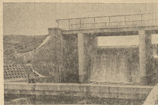
Przez granitowy jaz spadają wody jeziora sponad 4-metrowej wysokości, spływając trzema kaskadami w umocnione pusto-betami koryto odpływowe Cybiny. Na zdjęciu na pierwszym planie widoczny próg, który po zamknięciu dolnych prze-pustów spiętrzy wodę tworząc kaskadę.
