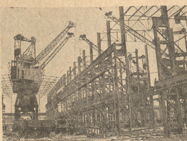
CAF — fot. Zyg. Wdowiński Budowa kombinatu hutniczego w Nowej Hucie postępuje szybko naprzód. Na zdjęciu: Fragment budowy jednej z wielu wielkich hal produkcyjnych
