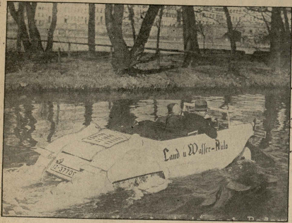
Niemiec Jakob Baulig w Koblenacji skonstruował samochód, który zarazem może być używany na wodzie jako motorówka.
