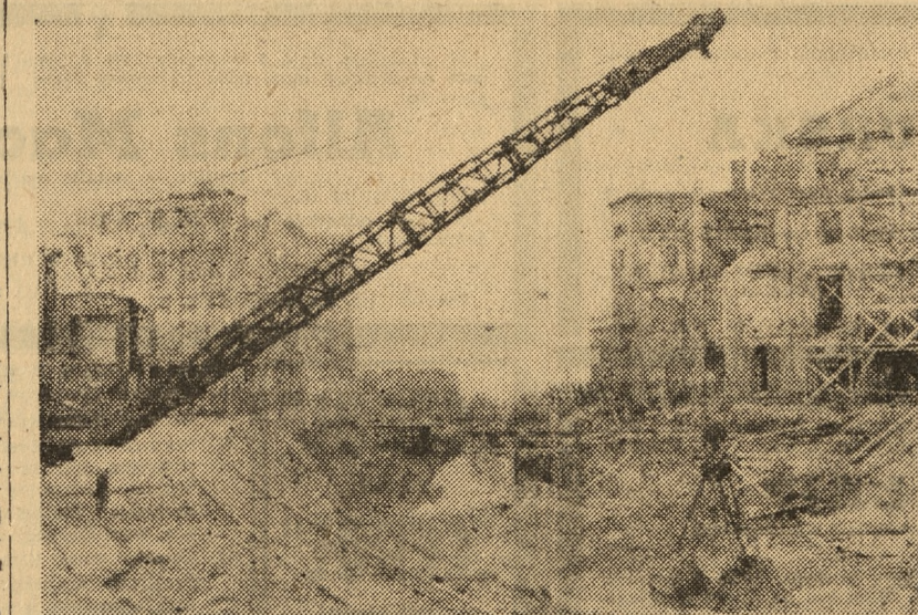
Na zdjęciu fragment prac przy tunelu wielkiej trasy komunikacyjnej Wschód — Zachód (pod placem Zamkowym i Krakow. Przedmieściem)
