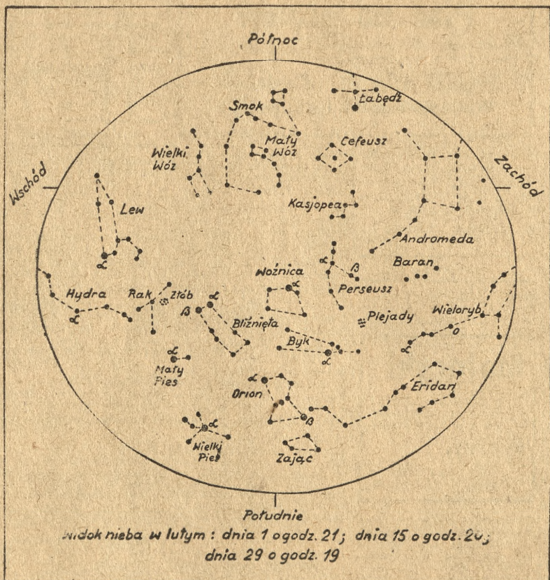
Mapka odpowiada wyglądowi nieba, gdy trzymamy ją ponad głową, odpowiednio zorientowaną względem stron świata. Kierunek północny znajdujemy, kierując się twarzą ku Gwiazdzie Biegunowej. Odnajdziemy ją, przedłużając 5-ciokrotnie odległość „tylnych kół” Wielkiego Wozu (Wielkiej Niedźwiedzicy).
