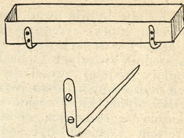
Sposób umocowywania skrzynki na hakach.
