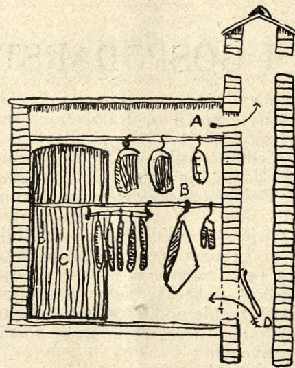
Wędzarnia na strychu, przybudowana do komina kuchennego.
