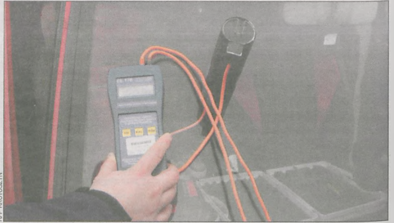
Urządzenie do pomiaru przepuszczalności światła w szybach pojazdów
