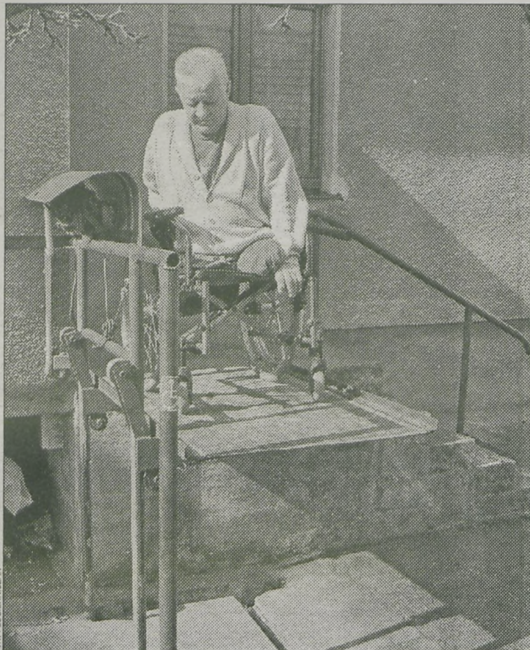
Andrzej Witczak, od czasu wypadku ponad 30 lat temu, jest inwalidą (nie ma nóg i jednej ręki). Mieszka w domku, który nie był przystosowany dla niepełnosprawnego. 7 lat temu sam zaprojektował i pomagał w budowie własnej windy, która do dzisiaj pozwala mu opuszczać samodzielnie mieszkanie.
