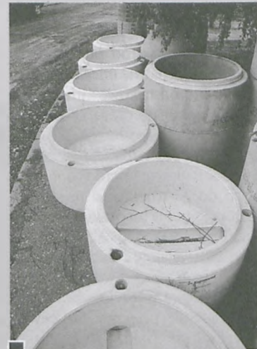
Pierwsze studzienki rewizyjne, które Aquanet montuje na poszczególnych posesjach przy ul. Krętej. Dzięki temu wszyscy będą podłączeni do sieci i nie będzie w przyszłości potrzeby cięcia asfaltu skanalizowania posesji fot. Piotr P. Ruszkowski
