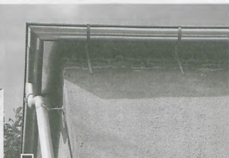
Skute gzymsy i wysunięte do ocieplenia: opierzenie i rynny fot. Piotr Paweł Ruszkowski
