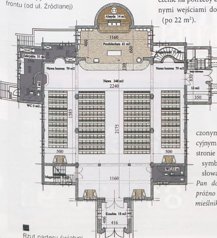
Rzut parteru świątyni
